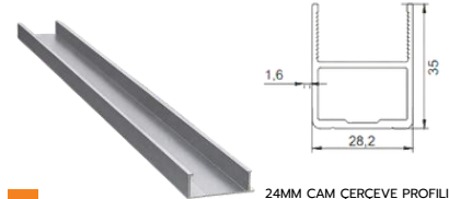
24MM CAM ÇERÇEVE PROFİLİ 24MM GLASS FRAME PROFILE
