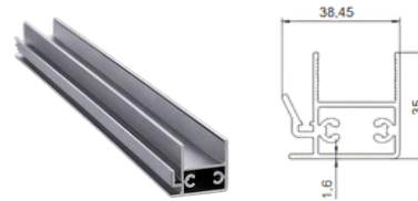
24MM CAM ÇEKİCİ PROFİLİ 24MM GLASS PULLER PROFILE
