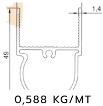
VASİSTAS MENTEŞE PROFİLİ TILT WINDOW HINGE PROFILE
