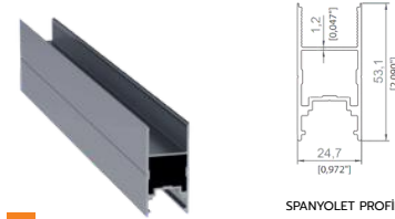
SPANYOLET PROFİLİ ESPAGNOLETTE PROFILE
