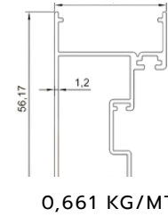
90 DERECE PROFİLİ 90-DEGREE PROFILE
