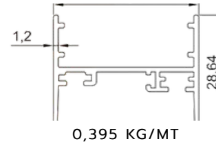
DÜZ ARKA DIŞI ÇITA PROFİLİ FLAT REAR FEMALE STRIP PROFILE
