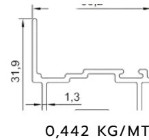
VASİSTAS ÇERÇEVE PROFİLİ TILT WINDOW FRAME PROFILE
