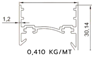
360 DERECE DIŞI AÇI PROFİLİ 360-DEGREE FEMALE ANGLE PROFILE
