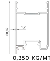
İSPANYOLET KİLİT PROFİLİ ESPAGNOLETTE LOCK PROFILE
