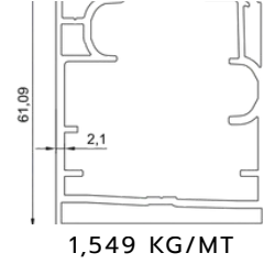
ALT-ÜST KASA PROFİLİ TOP & BOTTOM FRAME PROFILE
