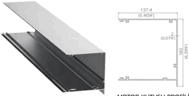
MOTOR KUTUSU PROFİLİ MOTOR BOX PROFILE
