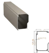
Motor Kutusu Profili Motor Box Profile
