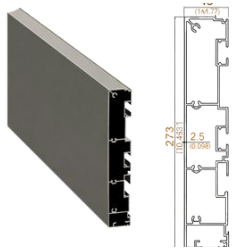
Oluk Dikme Profili Gutter Beam Profile
