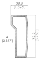
38,8x95,5 Oluk Eki Profili 38,8x95,5 Gutter Profile Connection
