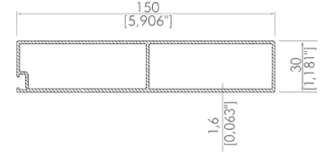
30x150 Kutu Profili 30x150 Box Profile
