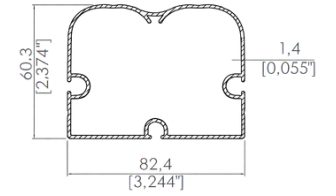
82,4x60,3 Kalın Korniş 82,4x60,3 Fabric Support Profile
