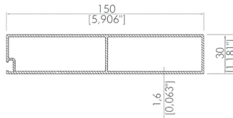
30x150 Kutu Profili 30x150 Box Profile
