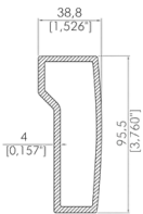
38,8x95,5 Oluk Eki Profili 38,8x95,5 Gutter Profile Connection
