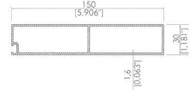
30x150 Kutu Profili 30x150 Box Profile
