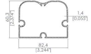
82,4x60,3 Kalın Korniş 82,4x60,3 Fabric Support Profile
