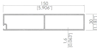
30x150 Kutu Profili 30x150 Box Profile
