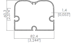
82,4x60,3 Kalın Korniş 82,4x60,3 Fabric Support Profile
